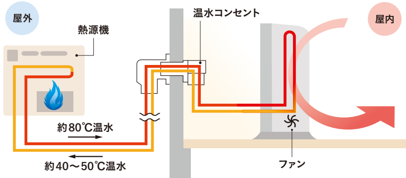
ガス温水ルームヒーターの仕組み
